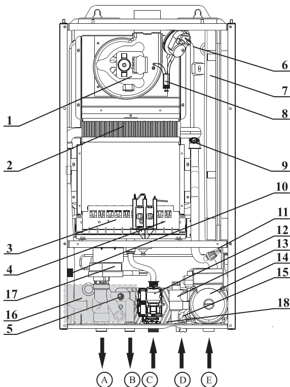
Котел ROYAL THERMO Aquarius MC (двухконтурный с отдельными теплообменниками)
