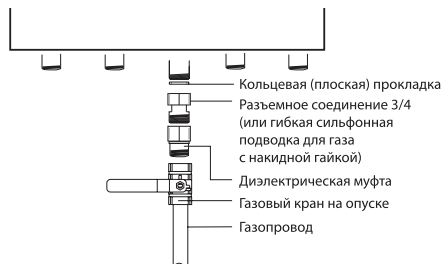
Подсоединение газопровод
